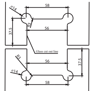
Kẹp xoay BHG 250
