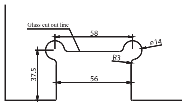
Kẹp xoay BHG 220
