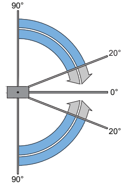
Reset area / Vùng giảm tốc độ
